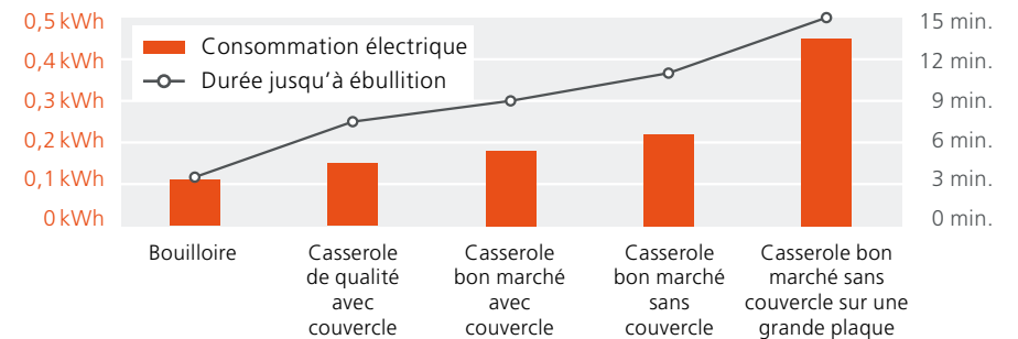
CONSOMMATION D'ÉLECTRICITÉ ET TEMPS NÉCESSAIRE POUR PORTER 1 LITRE D'EAU À ÉBULLITION
