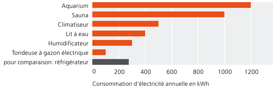
CONSOMMATIONS ÉLECTRIQUES ANNUELLES DES APPAREILS DE LA CATÉGORIE «DIVERS»
